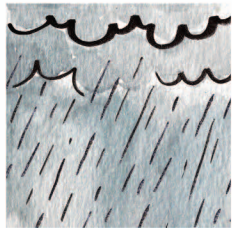
rain
